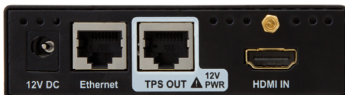
HDMI-TPS-TX95
